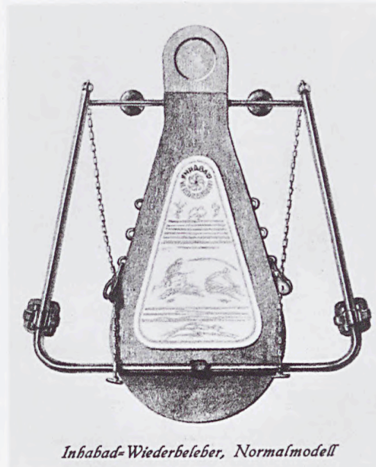
Reklamemarken der Inhabad GmbH Berlin und Abbildung des Inhabad-Apparats (ca. 1925), der die Handbeatmungsmethode nach Sylvester "ins Maschinelle übersetzte".
