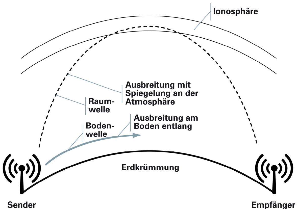
Abbildung: Ausbreitung einer elektromagnetischen Welle
