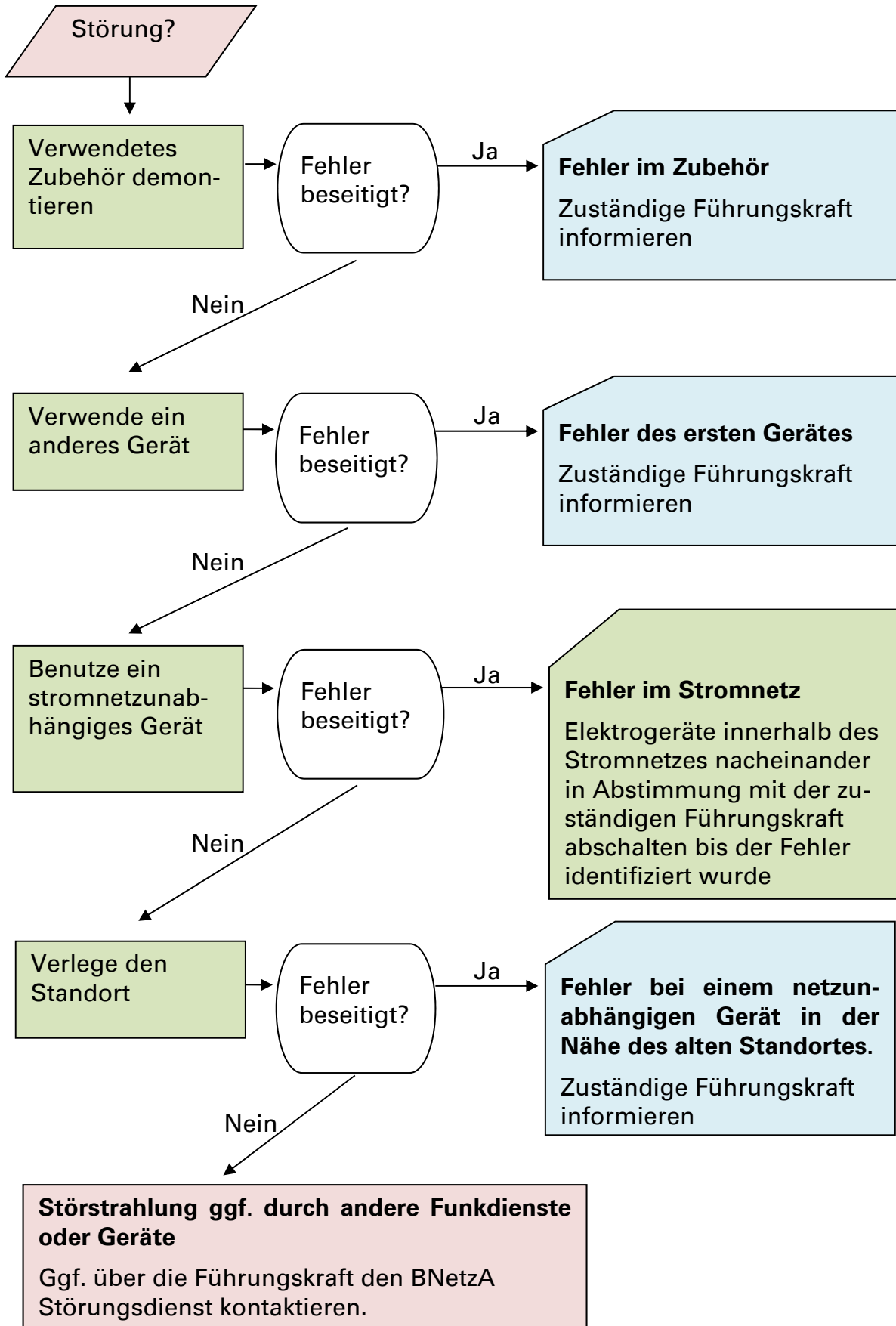
Abbildung: Störungsermittlung
