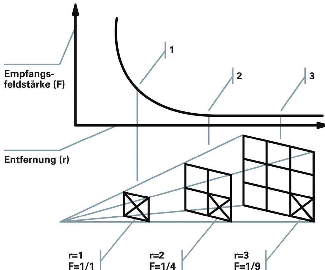
Abbildung: Empfangsfeldstärke
